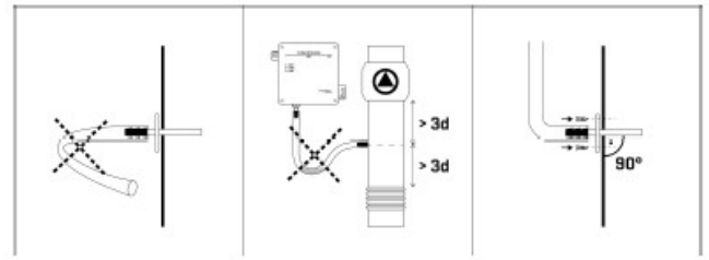
Rys. 3: Zalecenia montażowe
